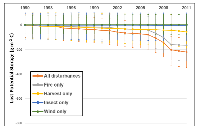
2.1d) Klamath National Forest
