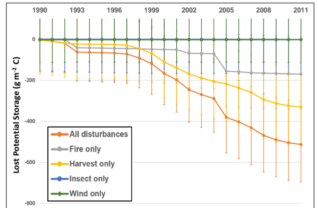
2.1b) Eldorado National Forest
