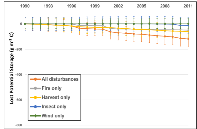
2.1h) Modoc National Forest
