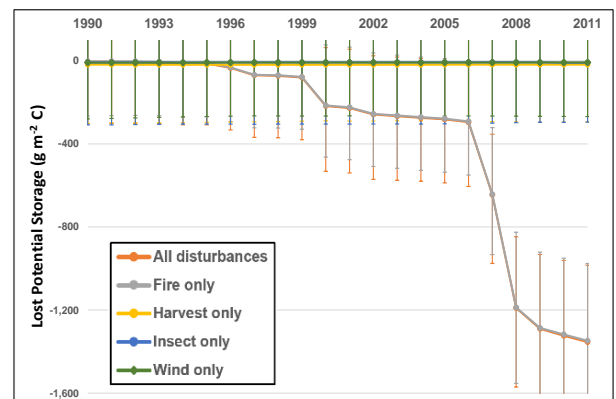
2.1f) Los Padres National Forest
